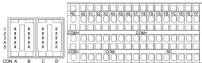
ユニットの正面から見た場合 A module view from the top
