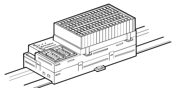
図 2.5 平面取り付け Fig. 2.5 Horizontal installation
