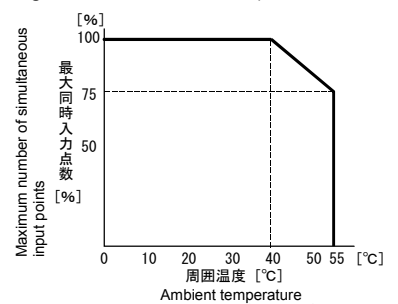
図 2.6 ディレーティングカーブ Fig. 2.6 Derating Chart
