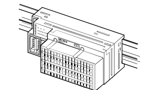
図 2.1 正面取り付け(正方向) Fig. 2.1 Front installation (Basic orientation)
